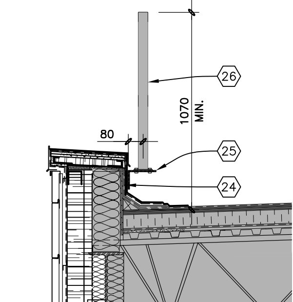
COUPE CONSTRUCTION
